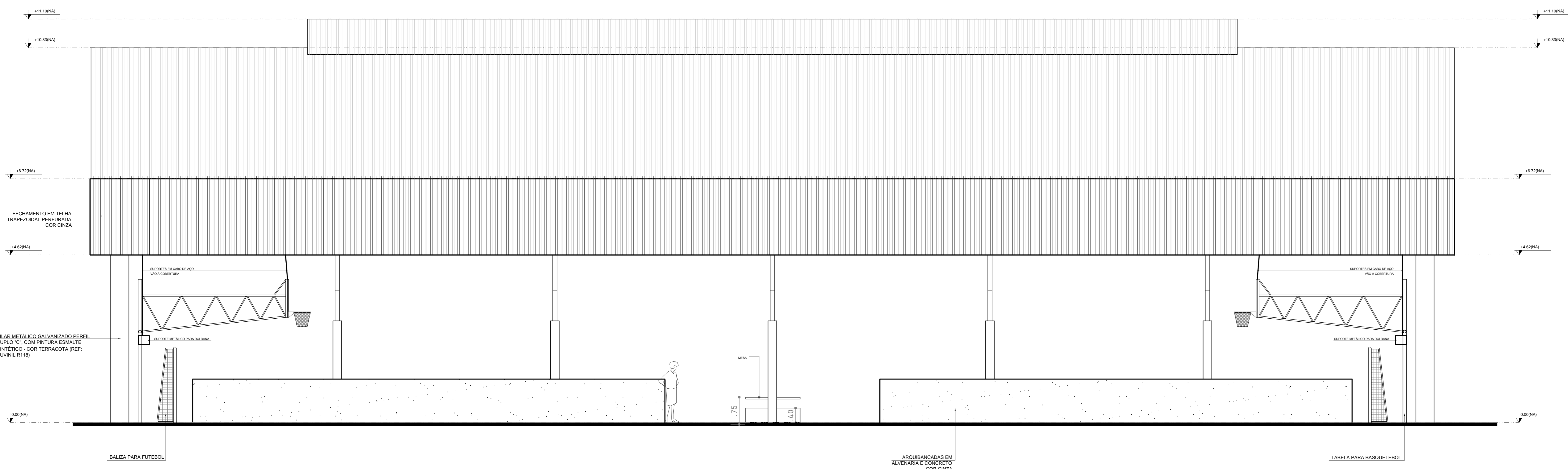
2 FACHADA 2 ESCALA 1/50
