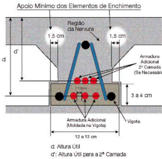
Nervura de lajes com vigotas treliçadas
