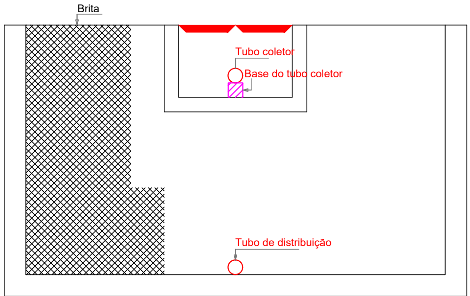
FILTRO ANAERÓBICO - Corte Escala 1/25
