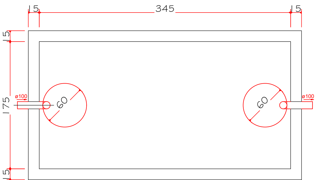
TANQUE SÉPTICO - Planta Baixa Escala 1/25
