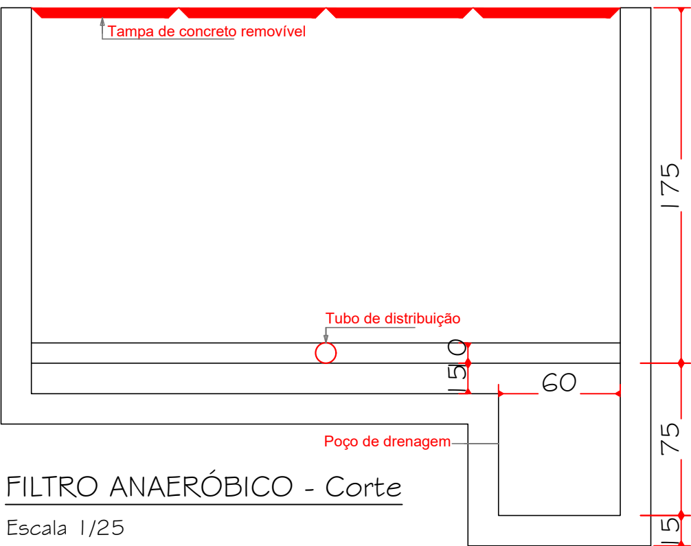
FILTRO ANAERÓBICO - Corte Escala 1/25
