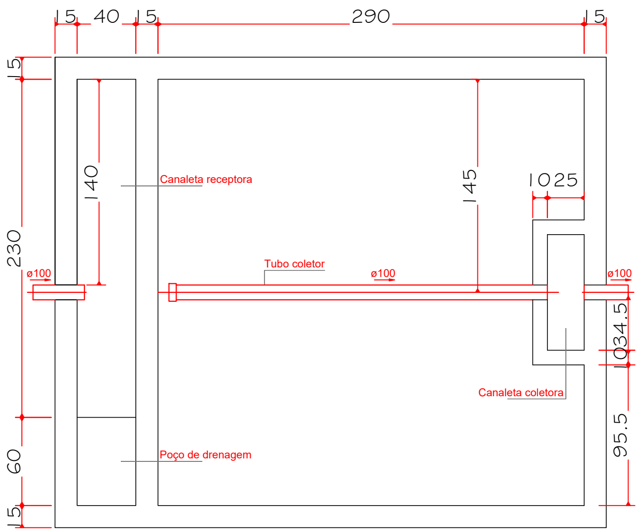
FILTRO ANAERÓBICO - Planta Baixa Escala 1/25
