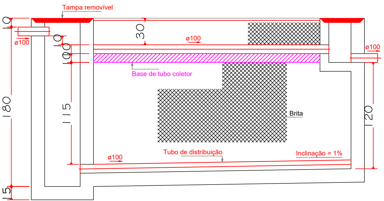
FILTRO ANAERÓBICO - Corte Escala 1/25
