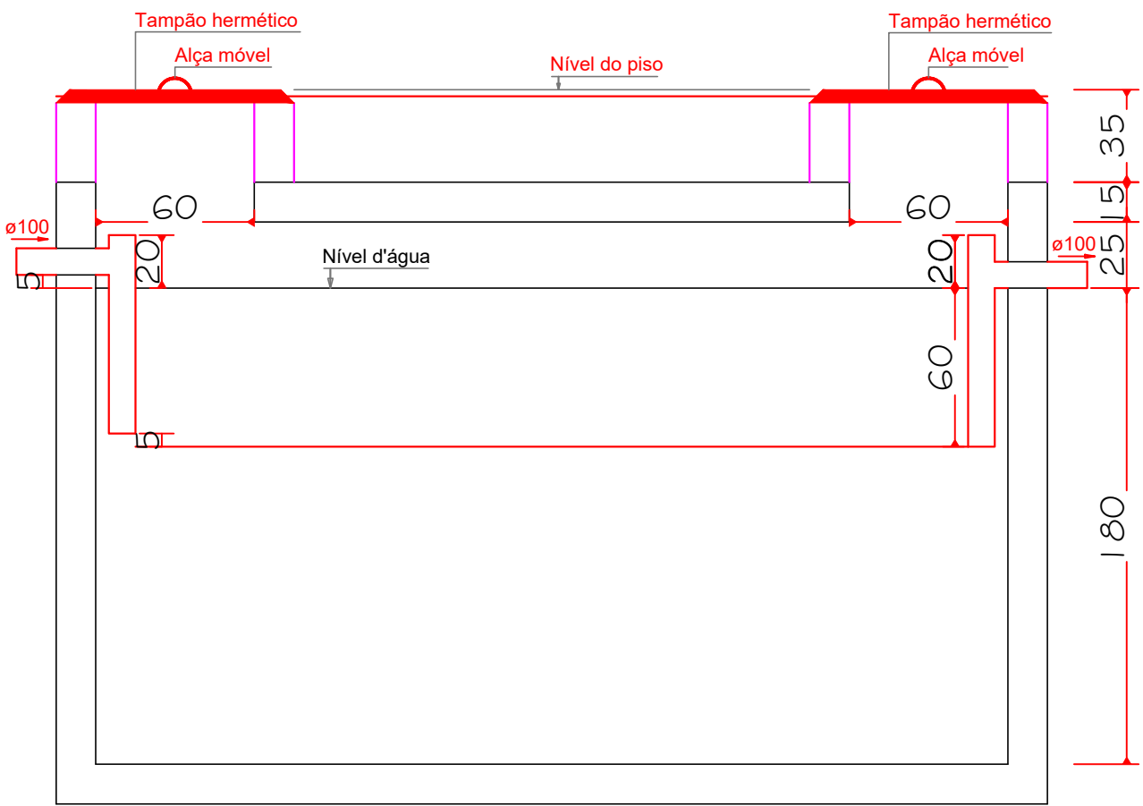
TANQUE SÉPTICO - Corte Escala 1/25
