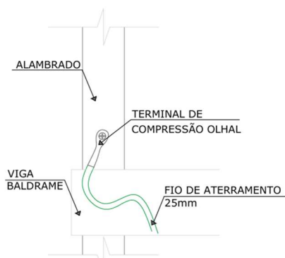
Figura 14– Detalhe de aterramento da quadra (Fonte: Autor/2025)
