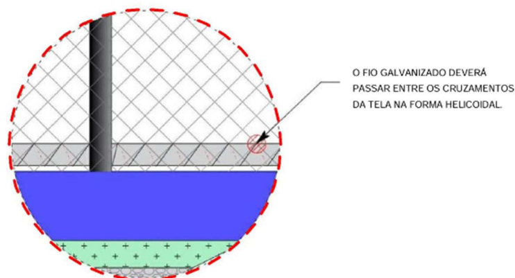
Figura 08 – Detalhe da fixação das telas (Fonte: Autor/2025)
