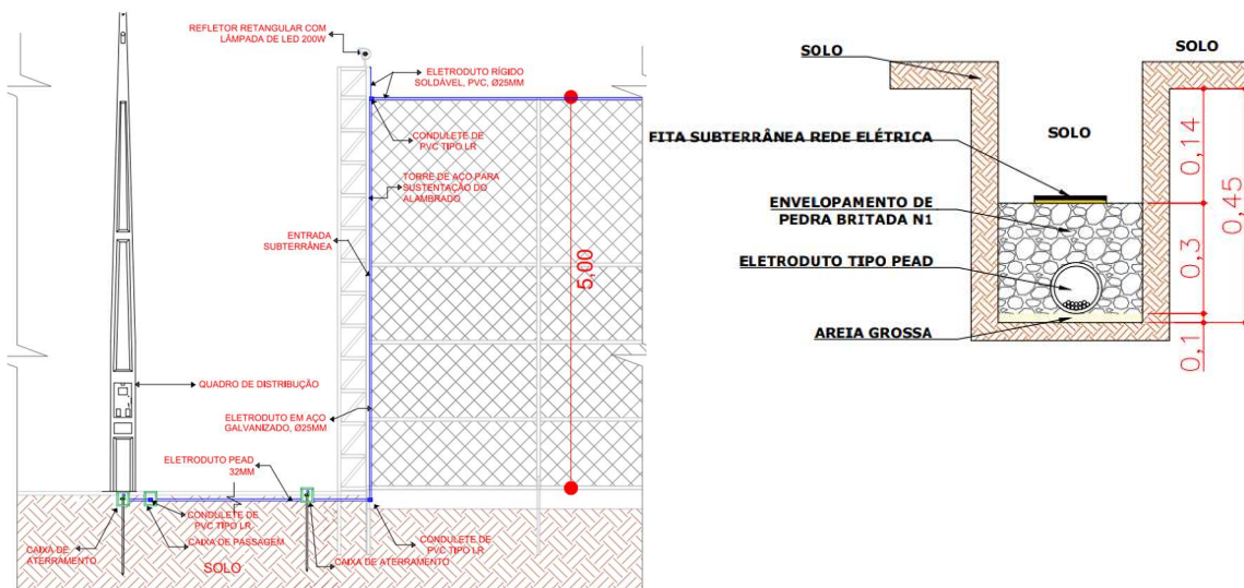
Figura 13 - Detalhes da elétrica (Fonte: Autor/2025)
