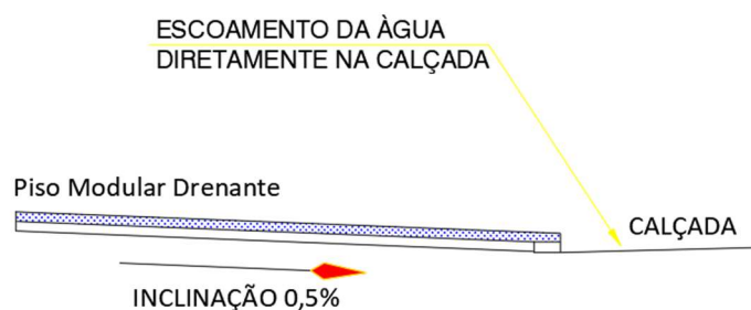
Figura 03 – Detalhe inclinação (Fonte: Autor/2025)
