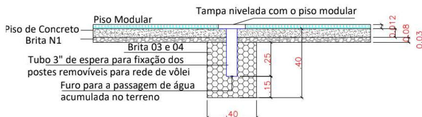
Figura 05 – Detalhe vala de drenagem espera do tubo da rede de vôlei (Fonte: Autor/2025)
