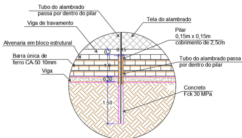
Figura 06 – Detalhamento de estaca (Fonte: Autor/2025)
