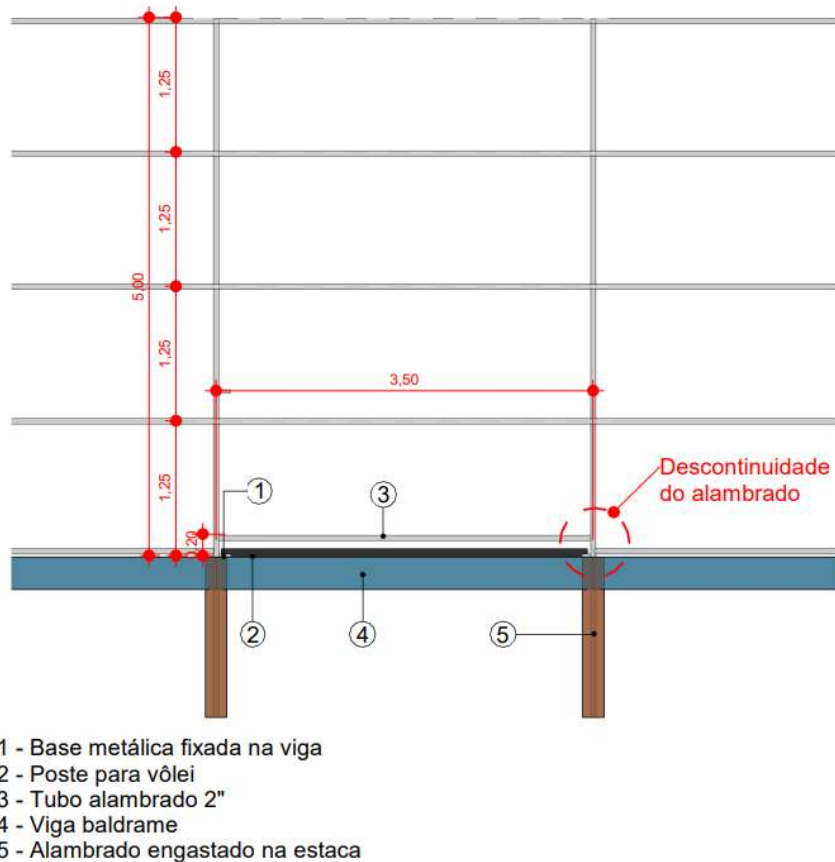
Figura 11 - Detalhe suporte para armazenamento do tubo de vôlei (Fonte: Autor/2025)
