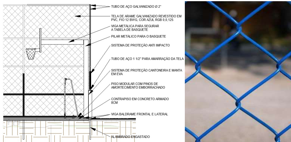
Figura 07 – Detalhe de alambrado (Fonte: Autor/2025)
