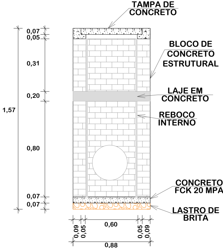
CORTE-BB
