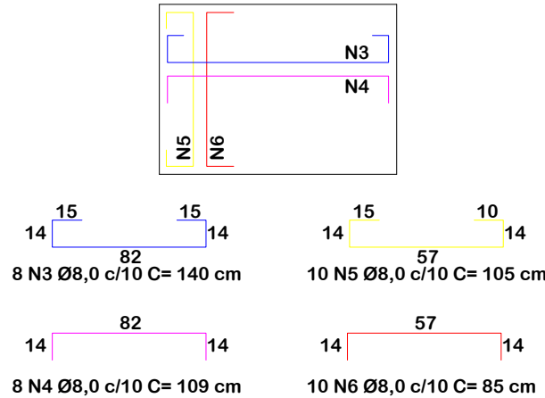
DETALHE DA LAJE
