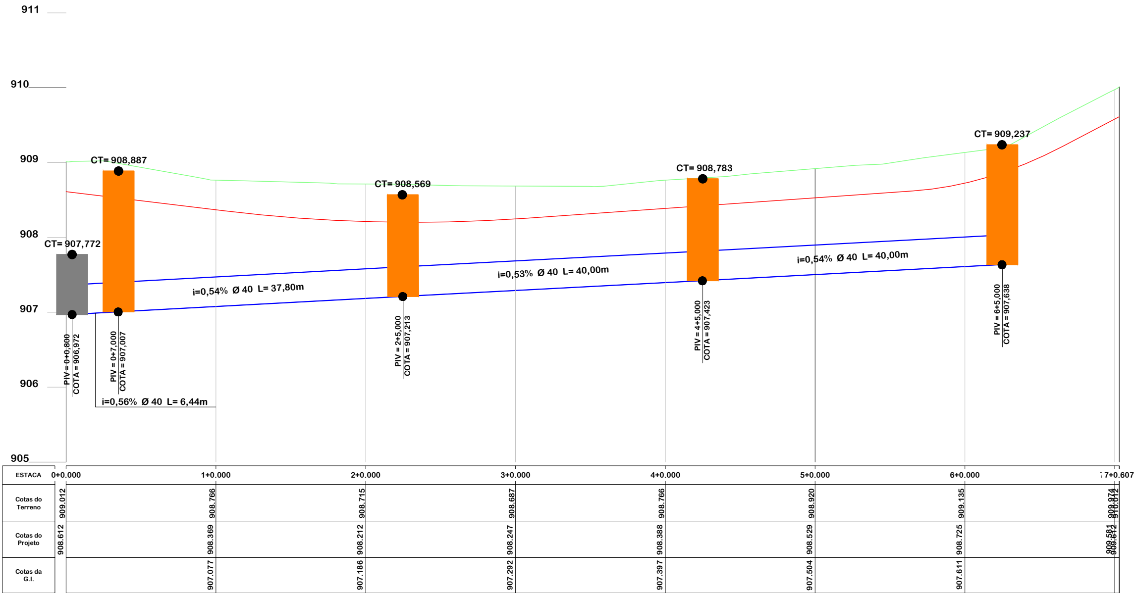
PERFIL LONGITUDINAL - LADO DIREITO
