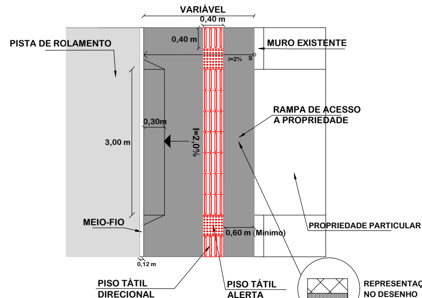
VISTA SUPERIOR - ACESSO A PROPRIEDADES PARTICULARES
