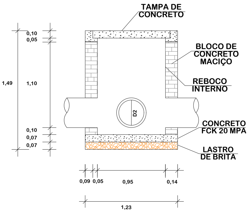
CORTE BB
