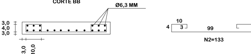
CORTE BB
