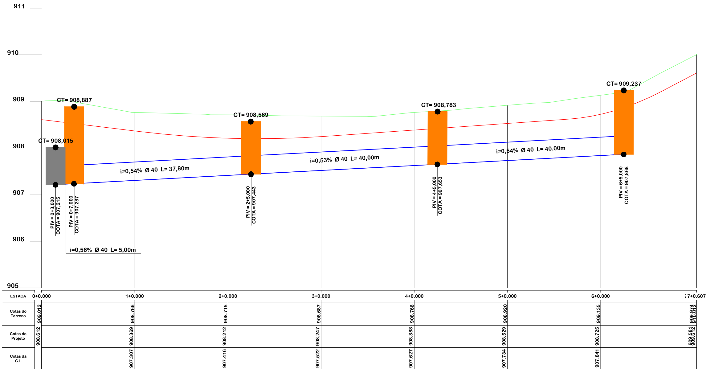
PERFIL LONGITUDINAL - LADO ESQUERDO
