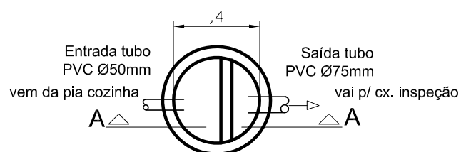
Planta Baixa
