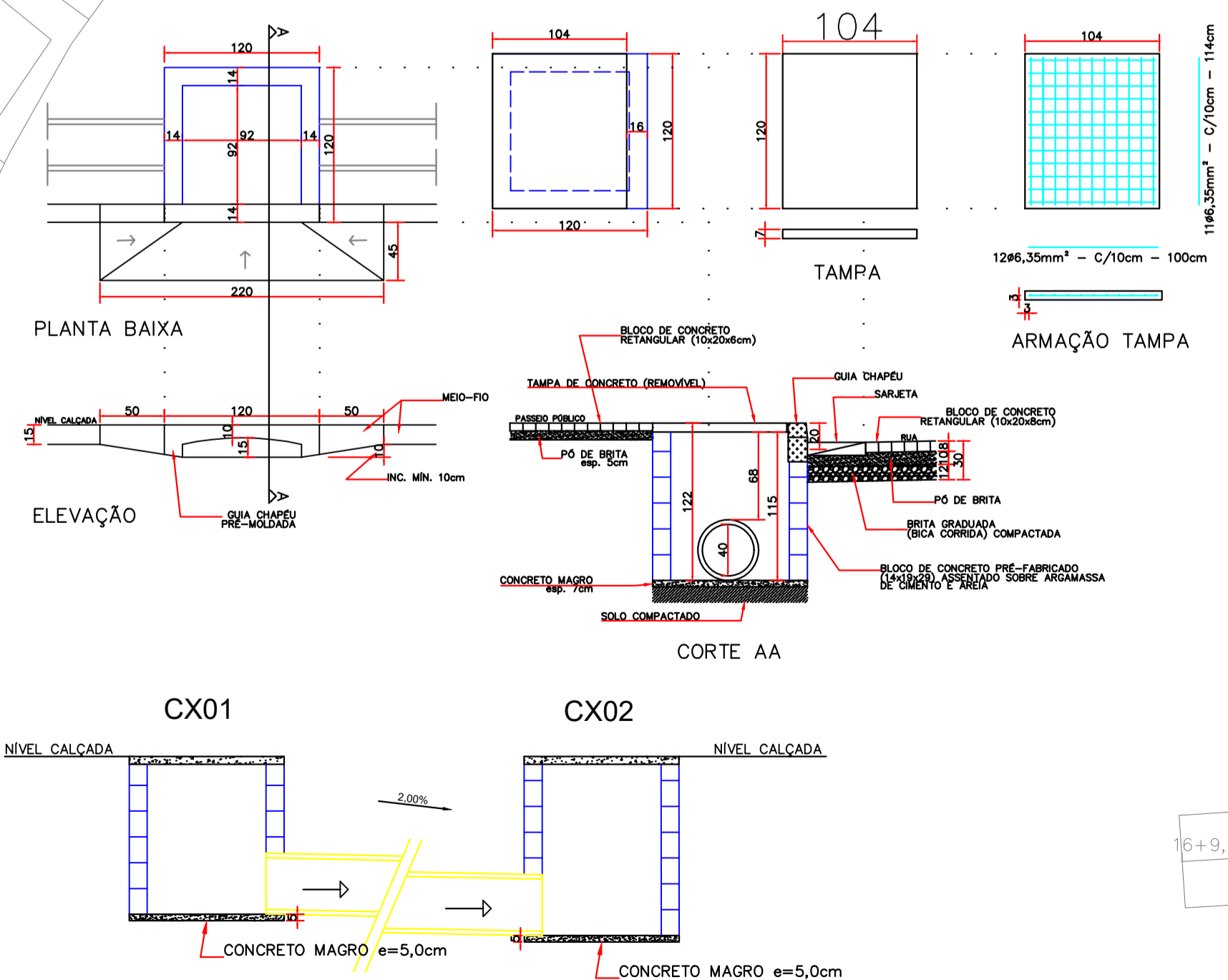
CAIXAS BOCA DE LOBO SIMPLES S/ESCALA
