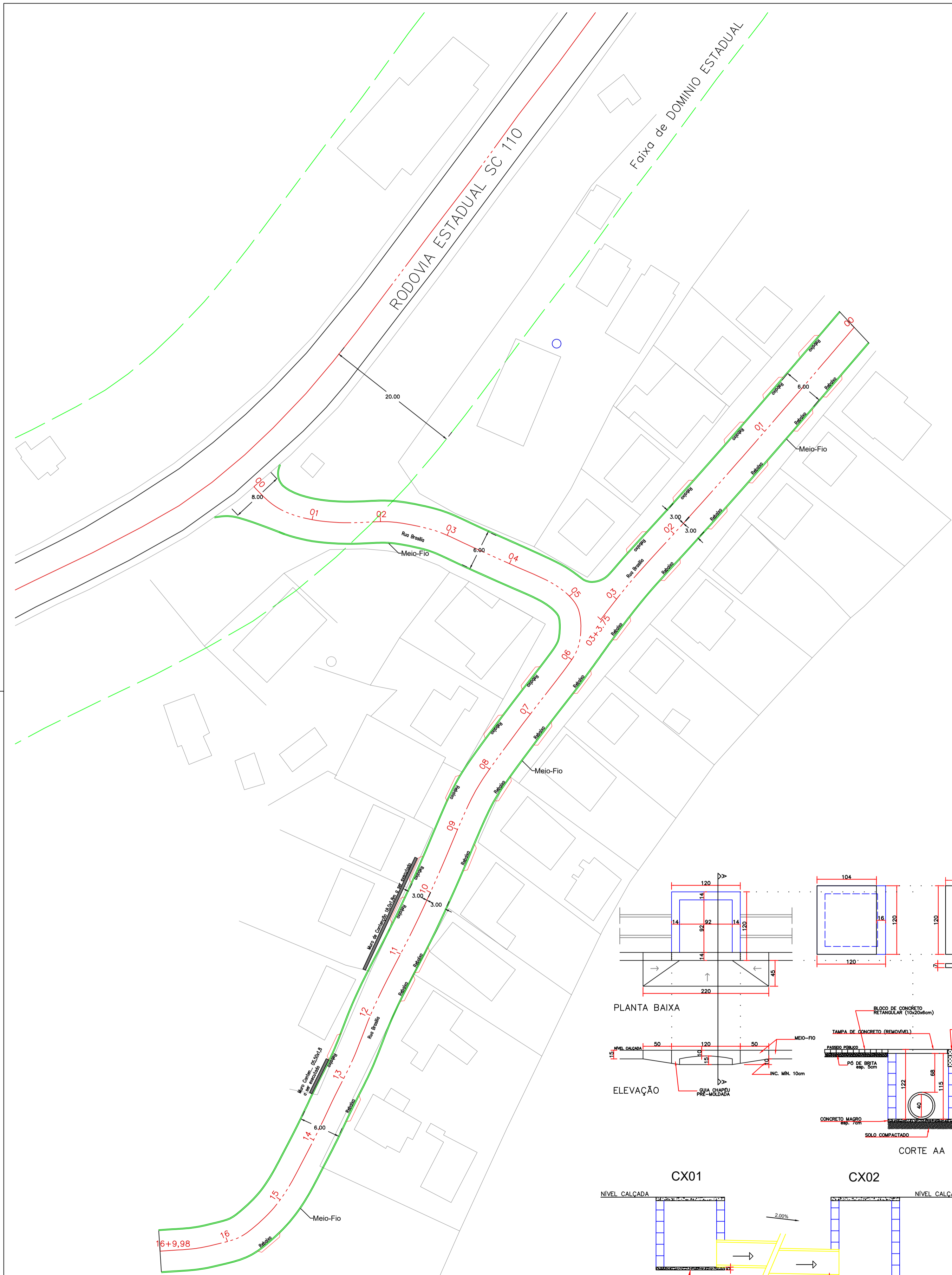
LOCAÇÃO ESC.: 1/300
