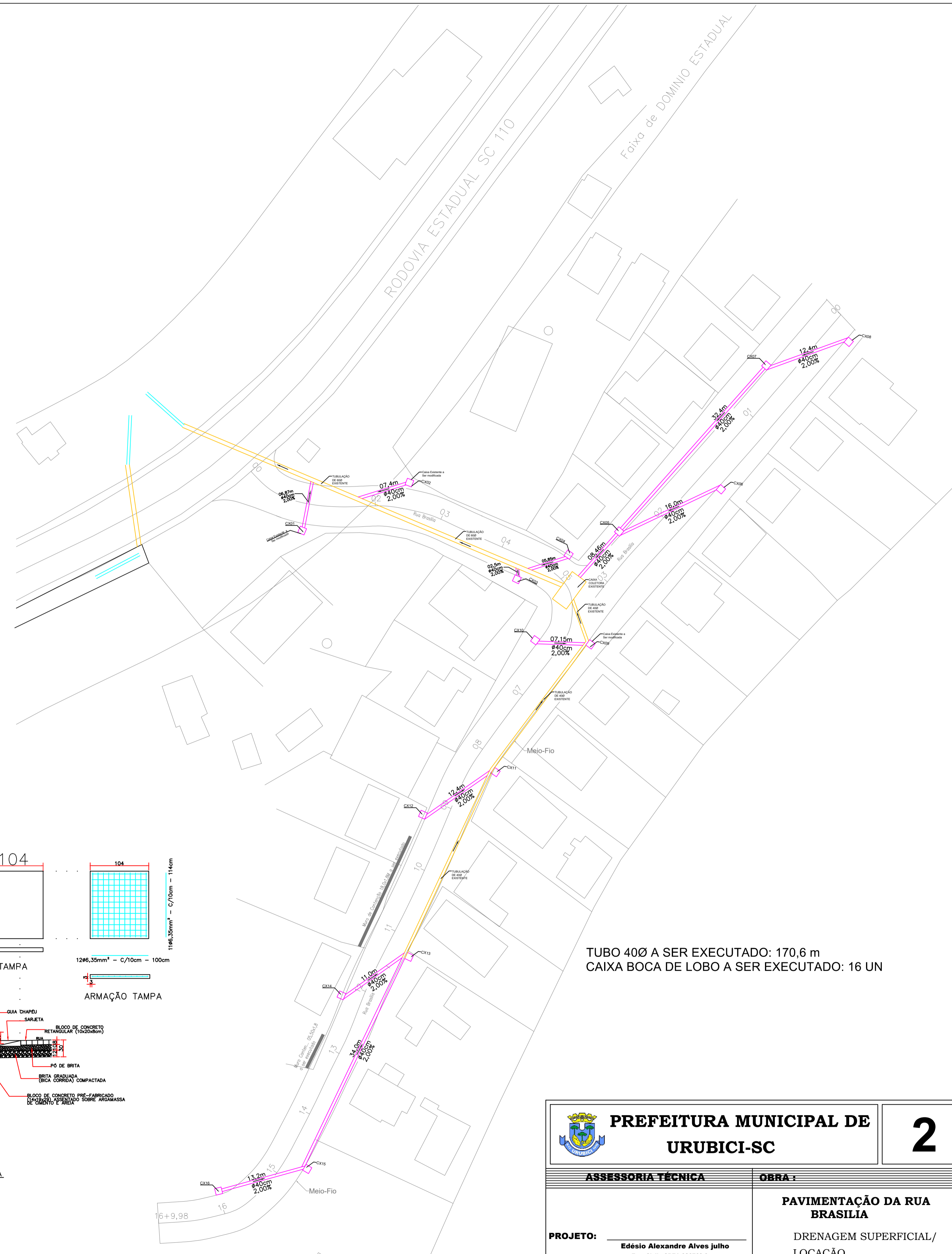
DRENAGEM SUPERFICIAL ESC.: 1/350
