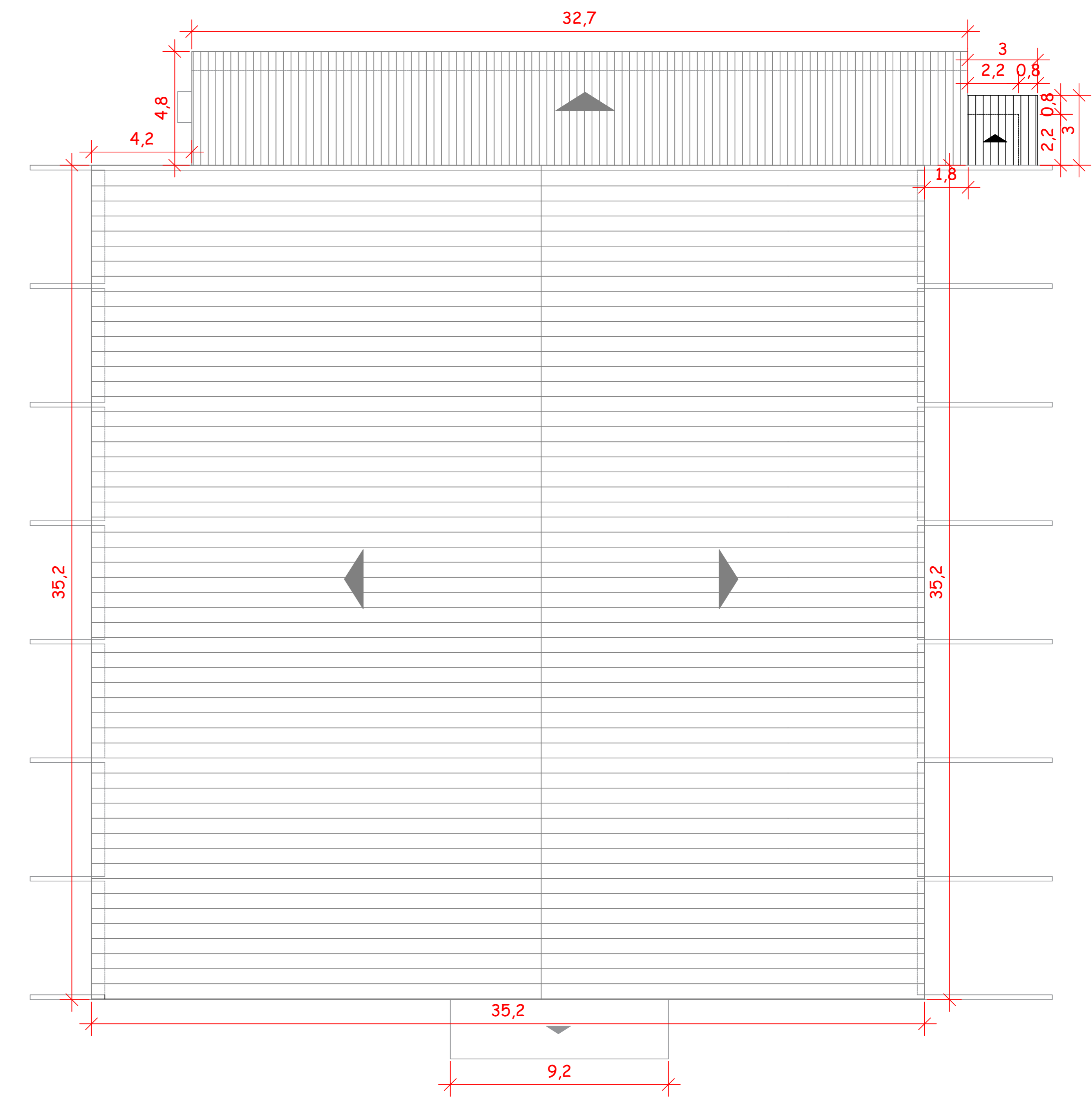
PLANTA DE COBERTURA ESC 1:125
